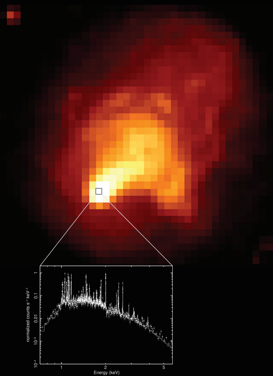
A2146. X-IFU. SIXTE
