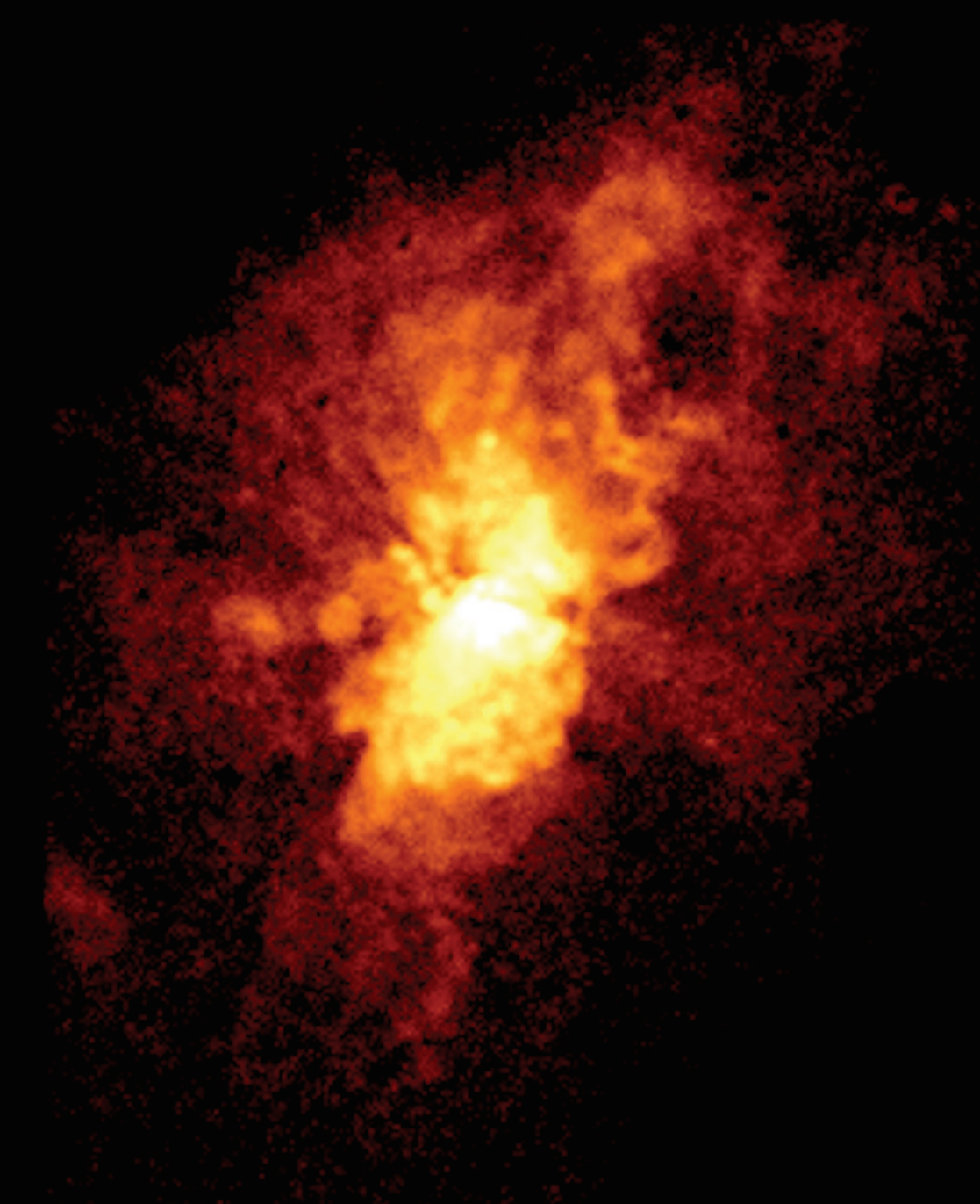
M82. WFI. SIXTE
